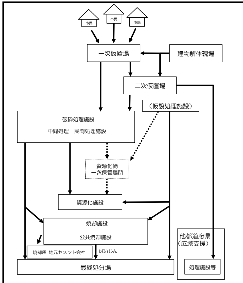
図表 1-14 災害廃棄物処理の流れ
