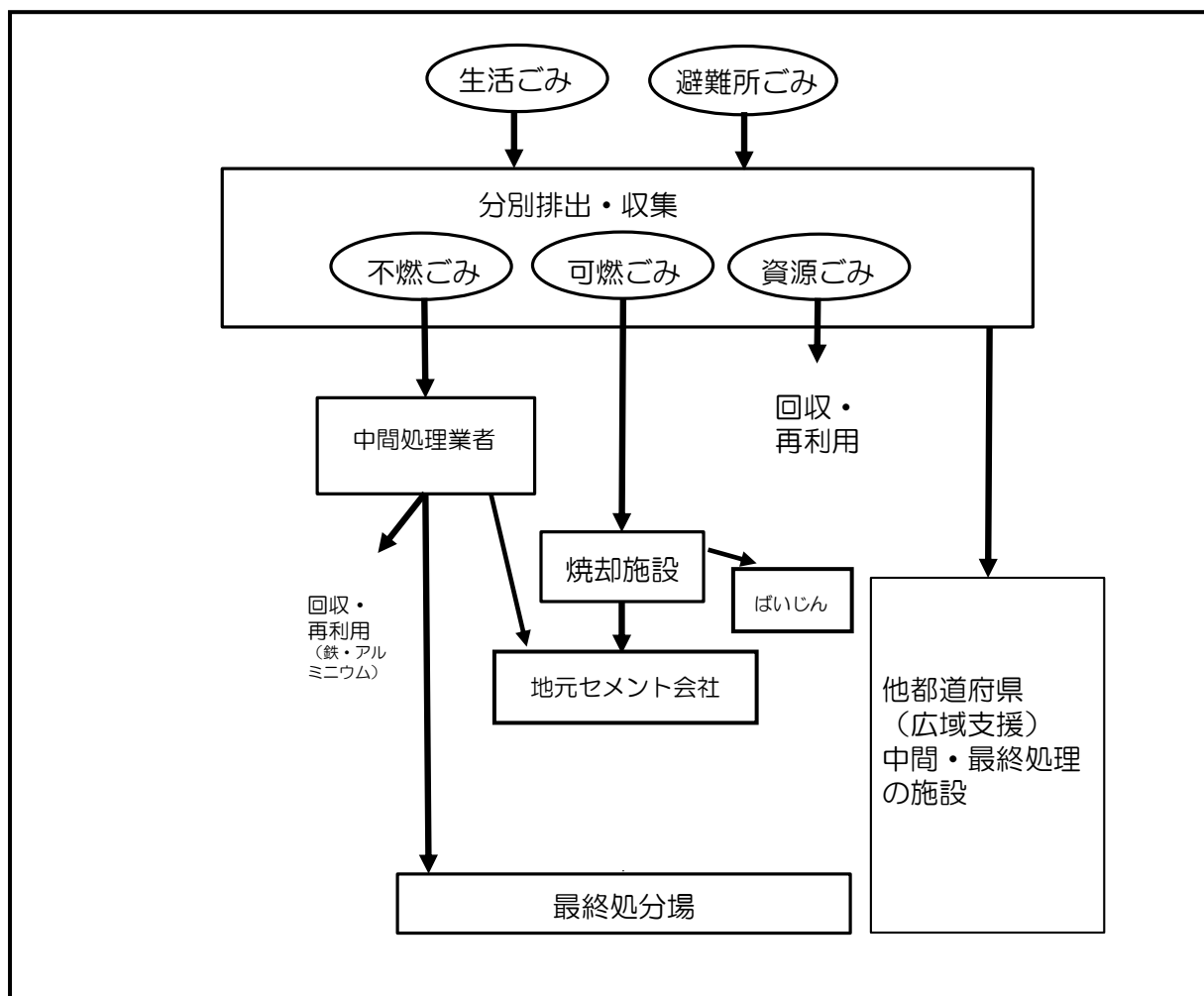
図表1-12 生活ごみ・避難所ごみの処理の流れ
